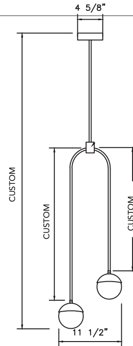
ELEVATION
